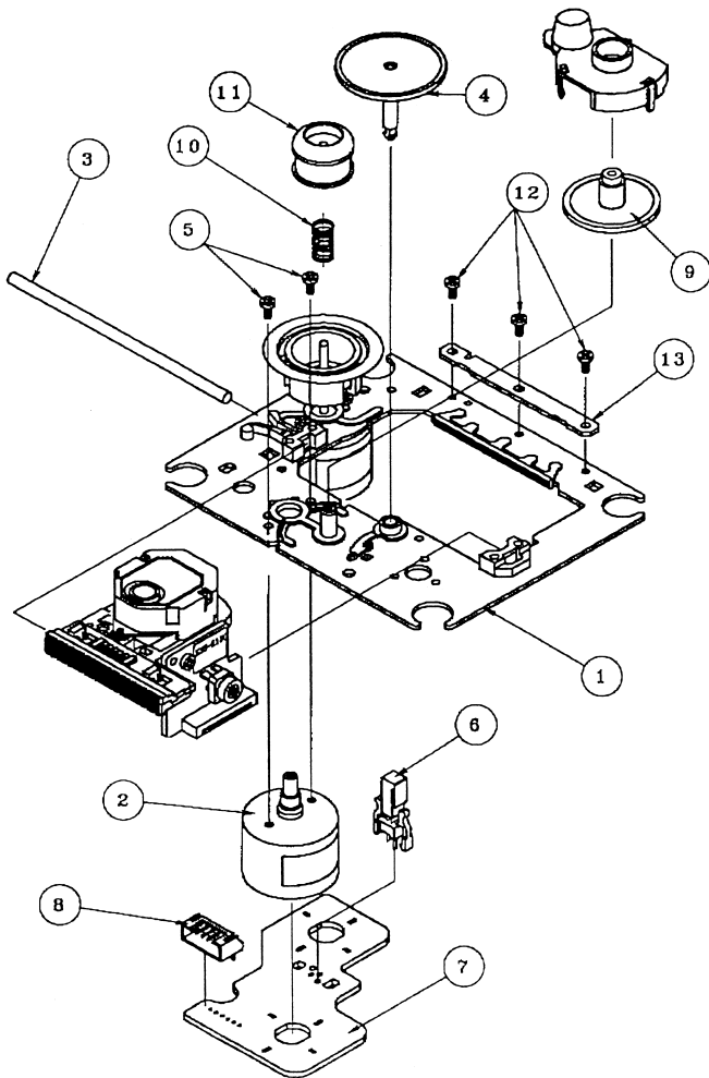
KSM-213CCM 分解図 Disassembly Drawing
