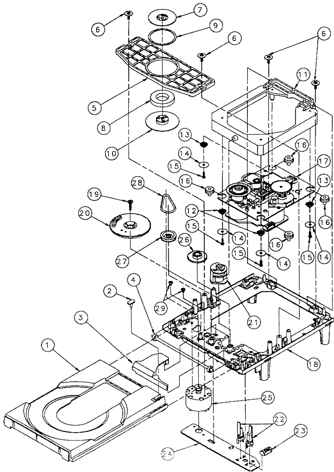
KSL-2130CCM 分解図 Disassembly Drawing
