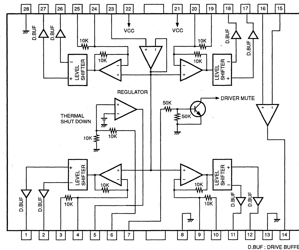
Fig. 9.9 Dirver BA6296FP
